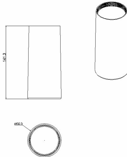
<Рис. 1.6.2.5 Размеры конуса 2 (140 мм)>
